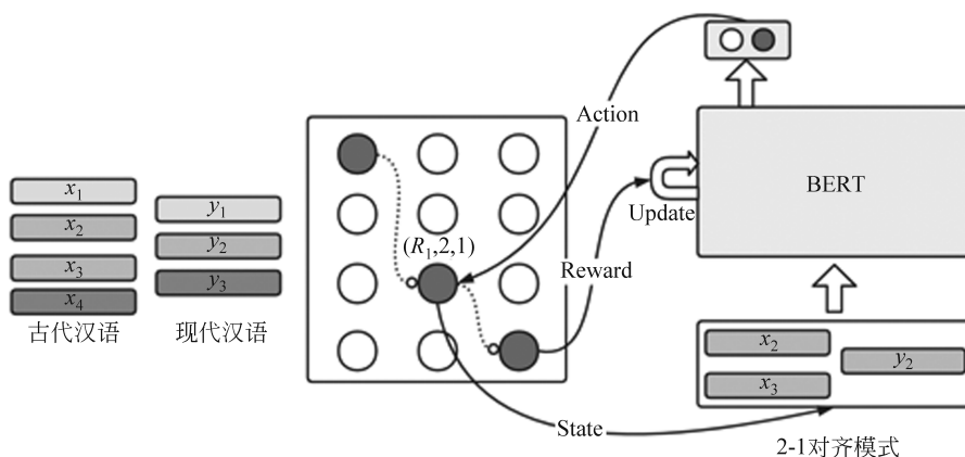
图 1 结合强化学习和预训练语言模型的策略网络模型
